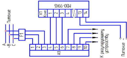
Ф1 – автомат защиты типа АК50Б-3М с током отсечки 5А; А1 – пускатель бесконтактный реверсивный ПБР-3А или усилитель тиристорный трехпозиционный ФЦ-0620
